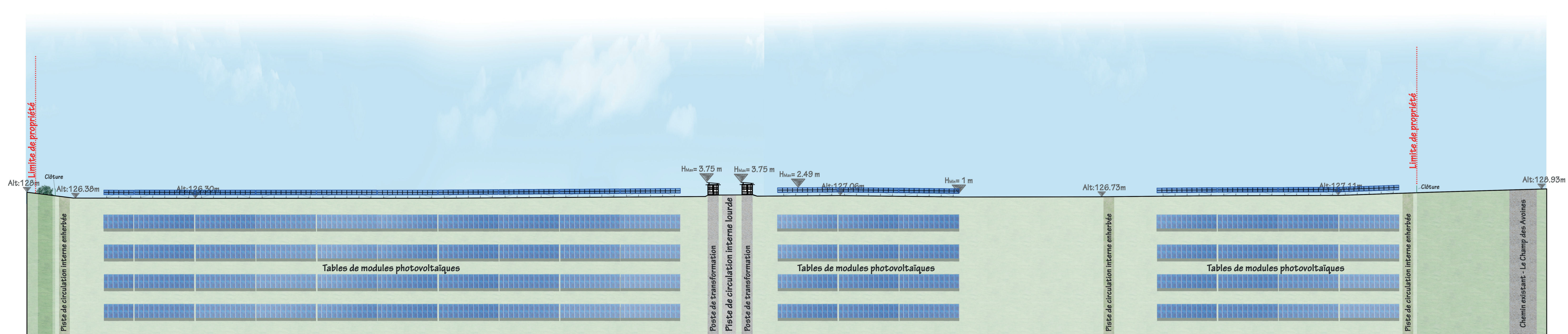
COUPE BB' : NORD / SUD DES PANNEAUX PHOTOVOLTAIQUES - échelle 1/500e
